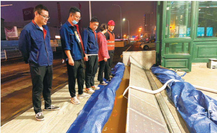
积水增多时,水动力全自动防洪闸可自行抬升阻水。
