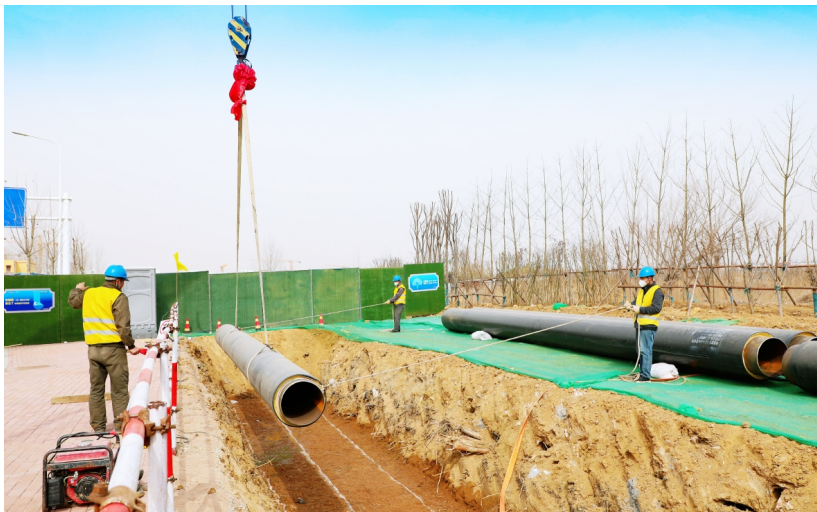
北部热源厂供热区域高温水替代蒸汽管线工程施工现场
